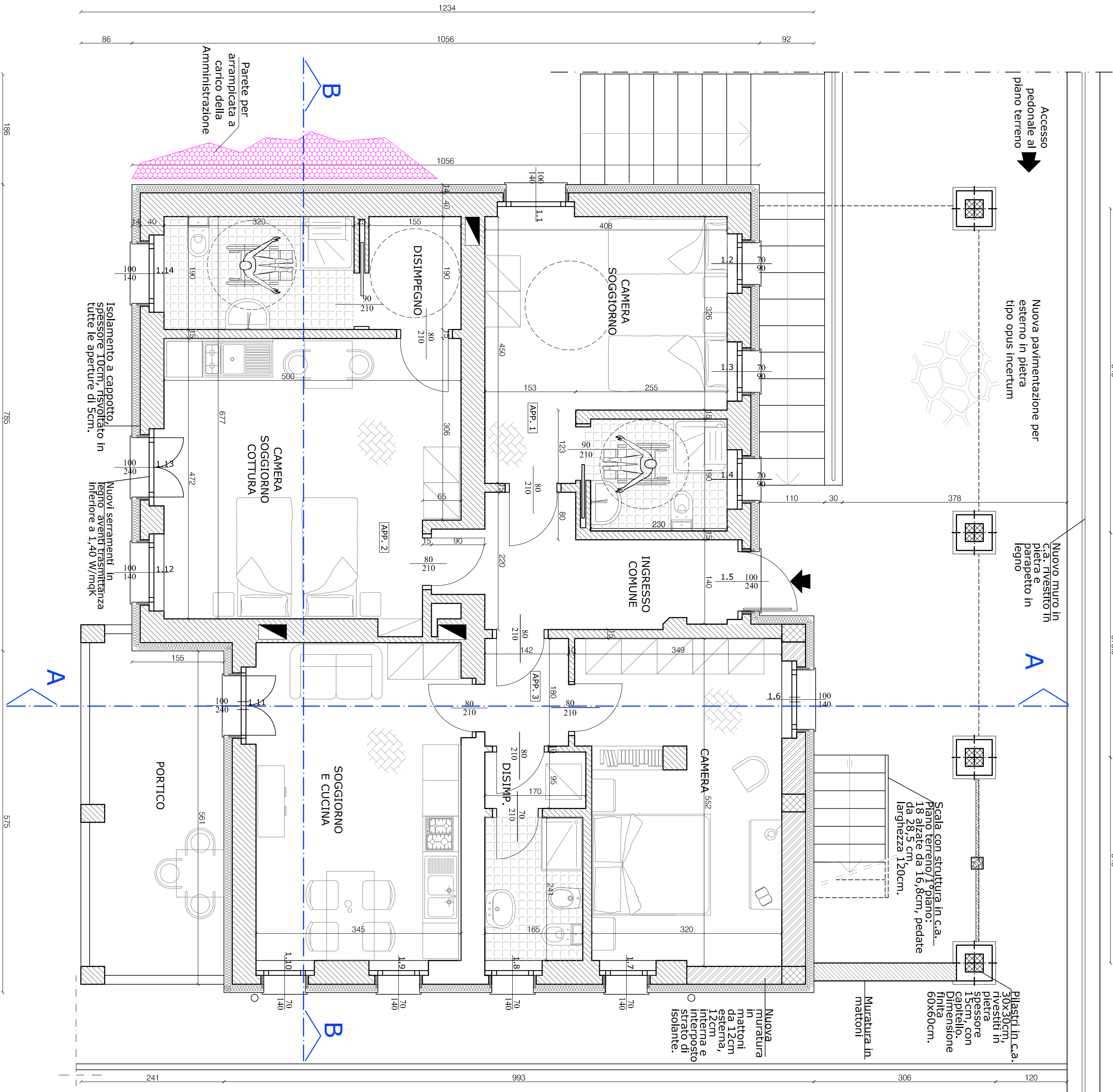
PIANO TERRENO - SCALA 1:50
