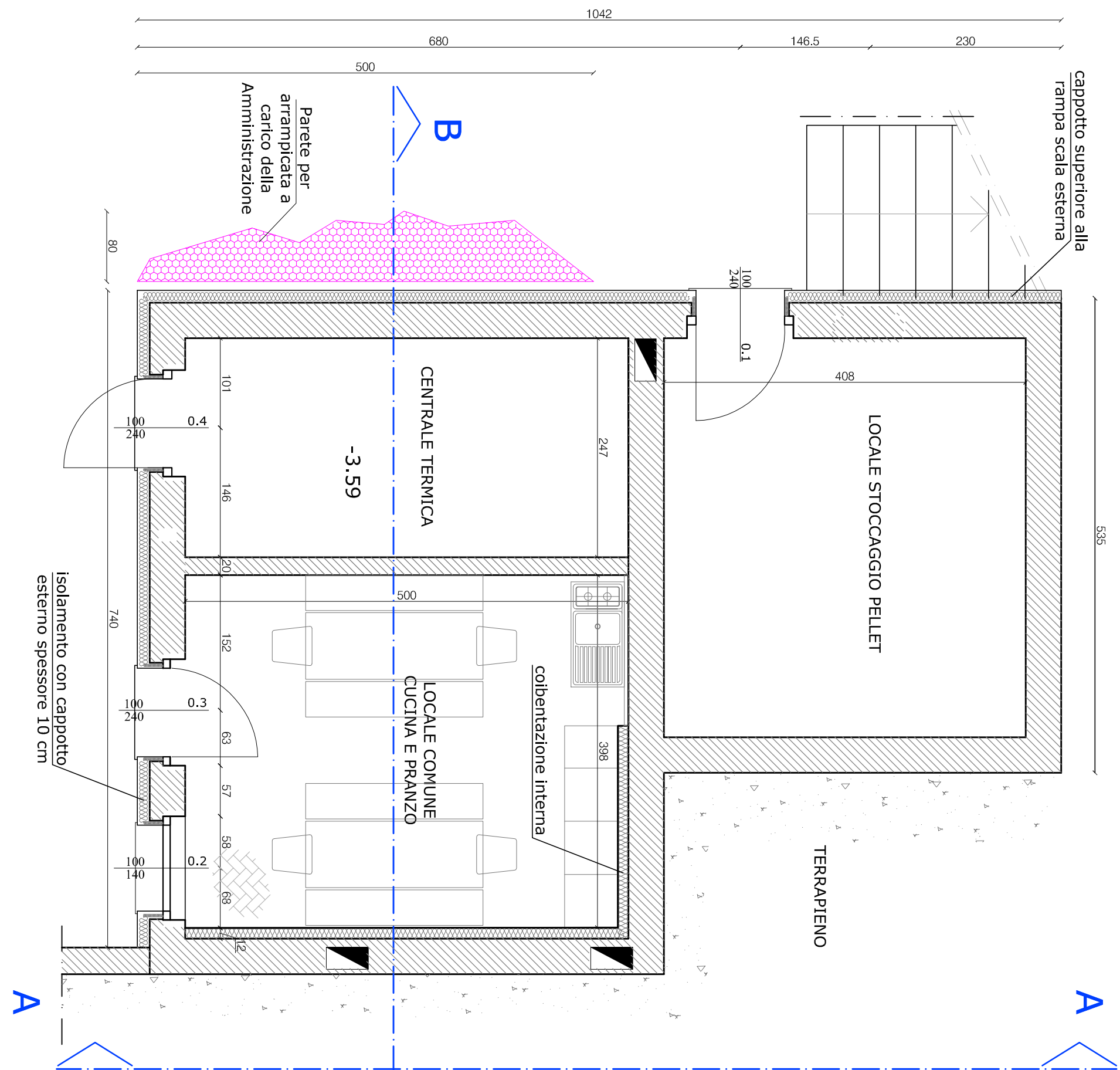
PIANO TERRENO - SCALA 1:50
