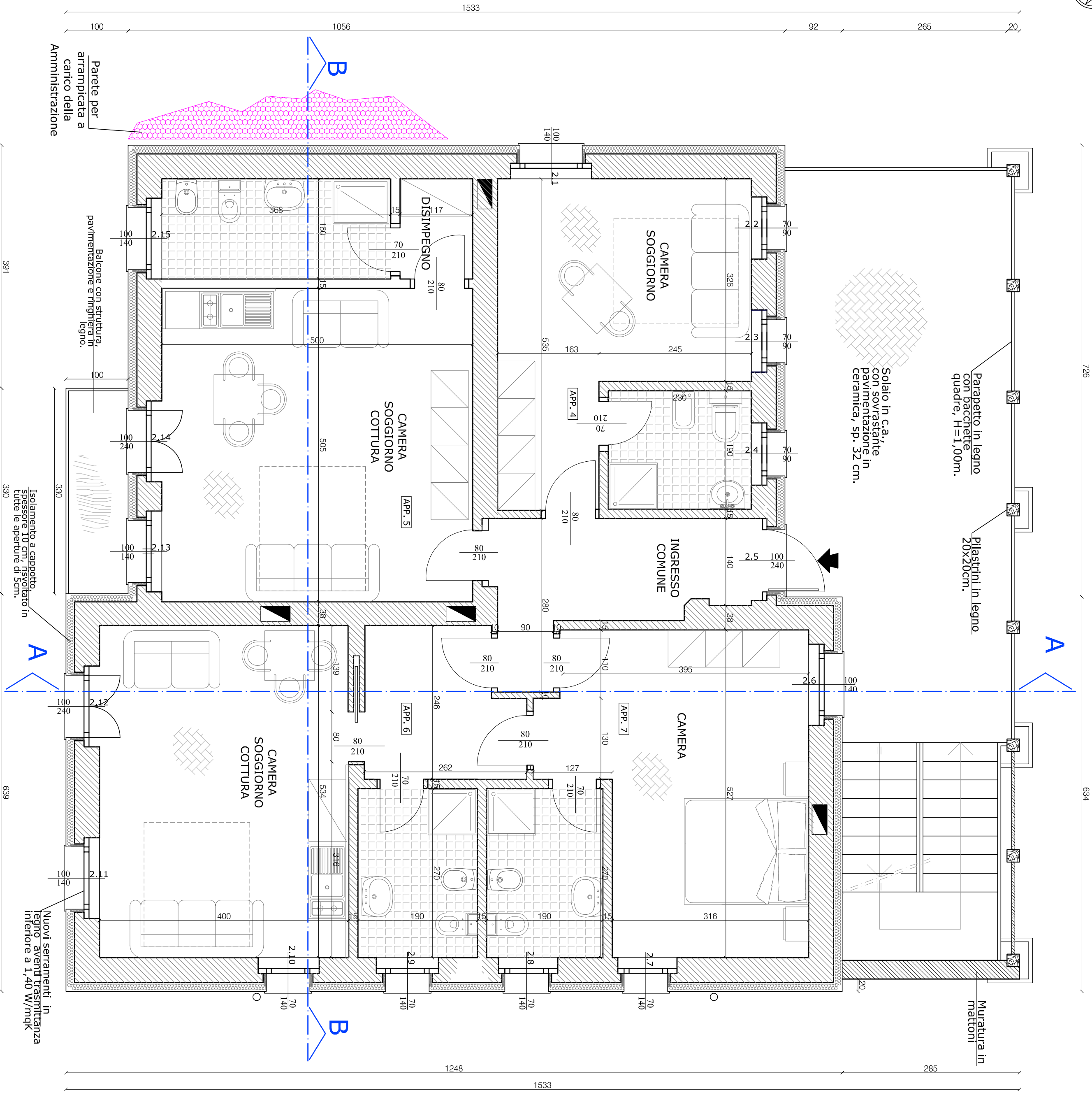
PIANO PRIMO - SCALA 1:50
