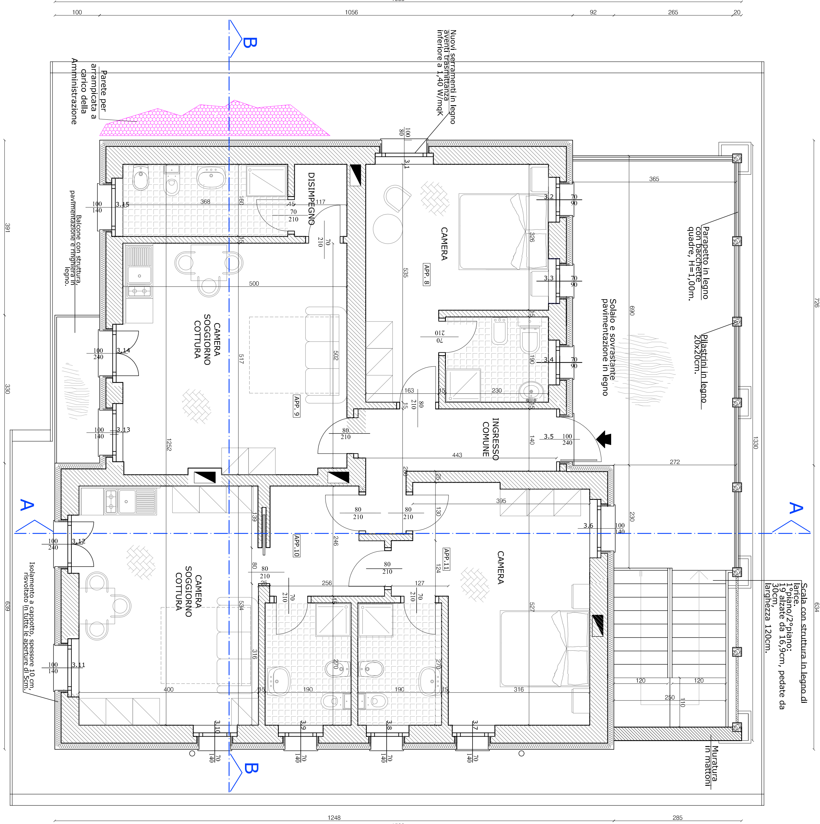
PIANO SOTTOTETTO - SCALA 1:50
