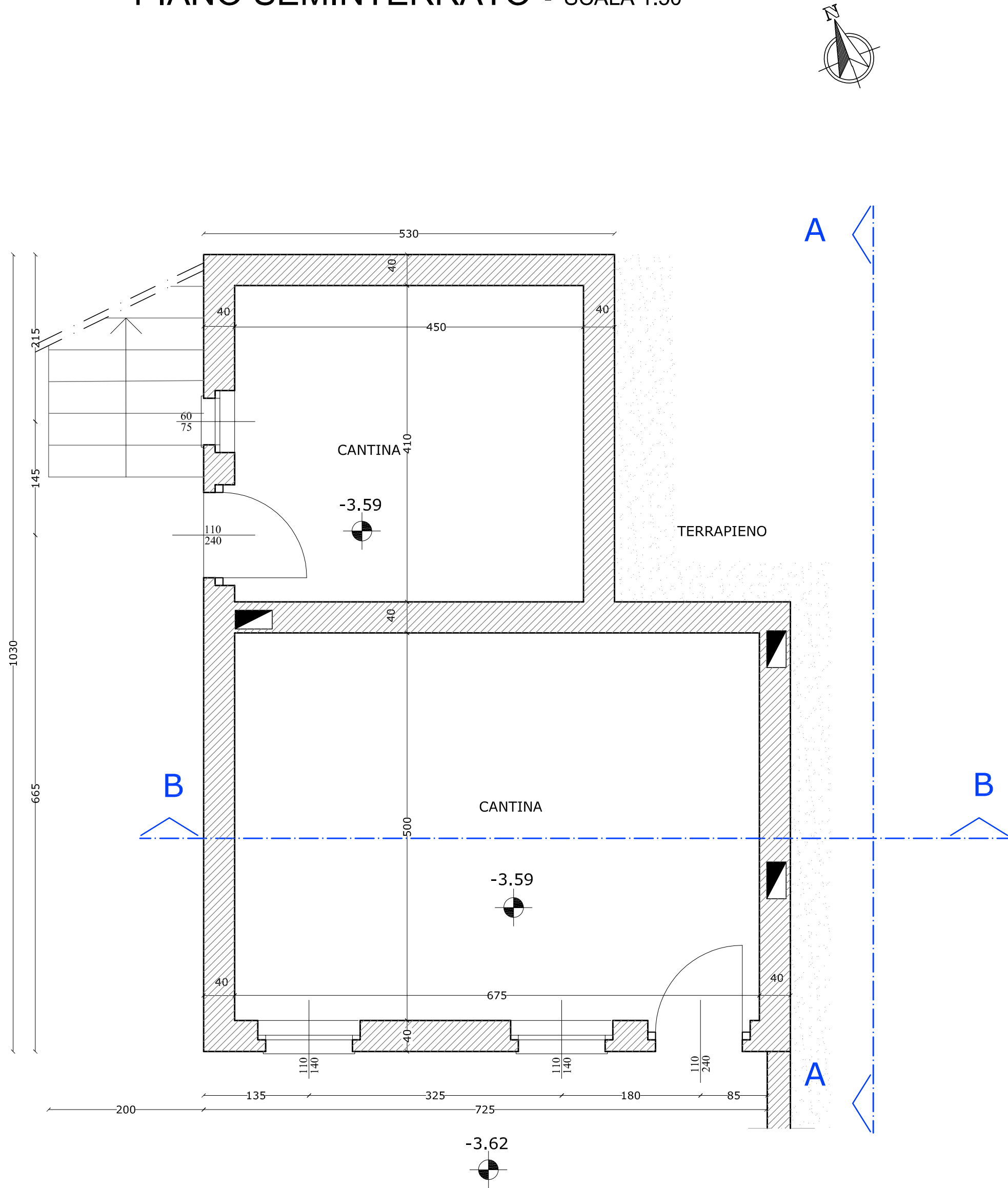
PIANO SEMINTERRATO - SCALA 1:50
