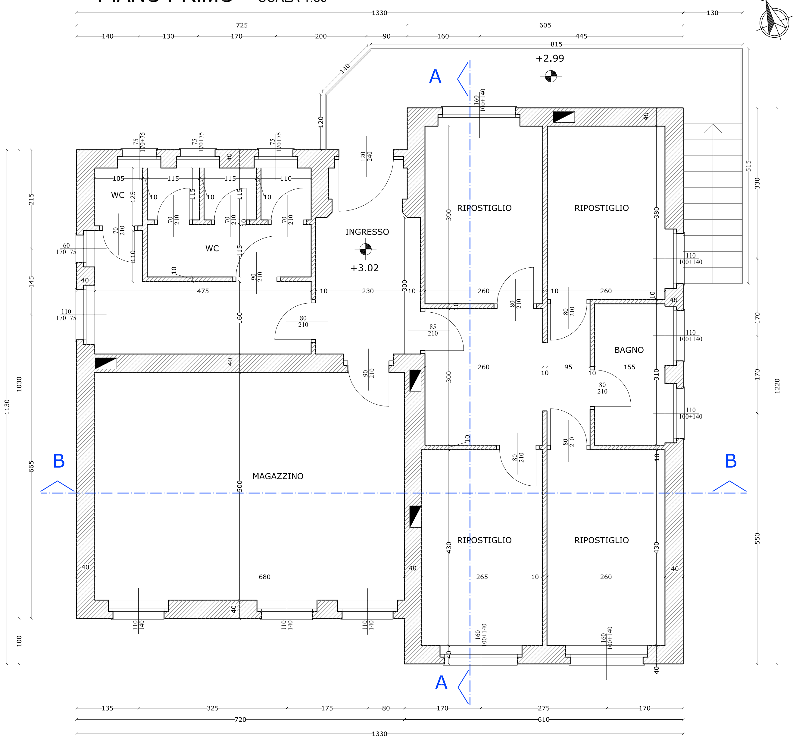
PIANO PRIMO - SCALA 1:50
